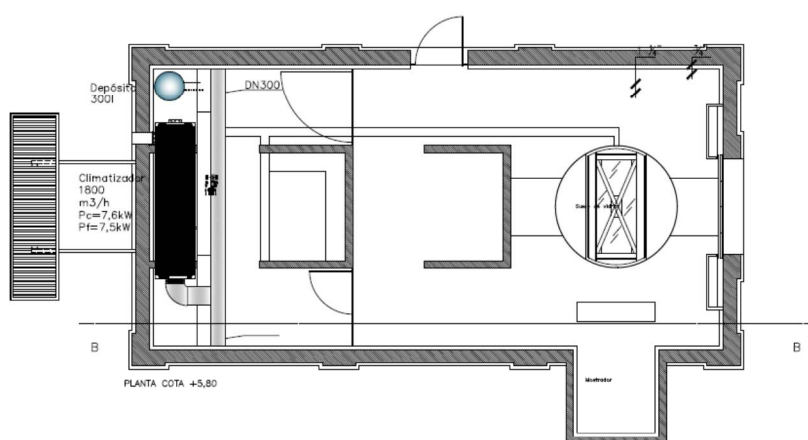
EDIFICIO RECEPCIÓN VISITAS SUP. APROX. 72 M 2
